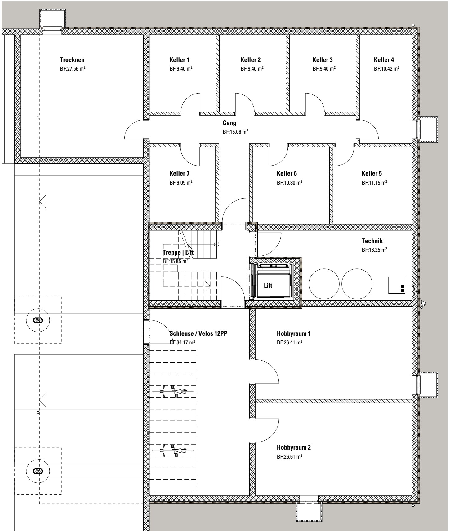
Haus B - UG - Keller / Hobbyräume
